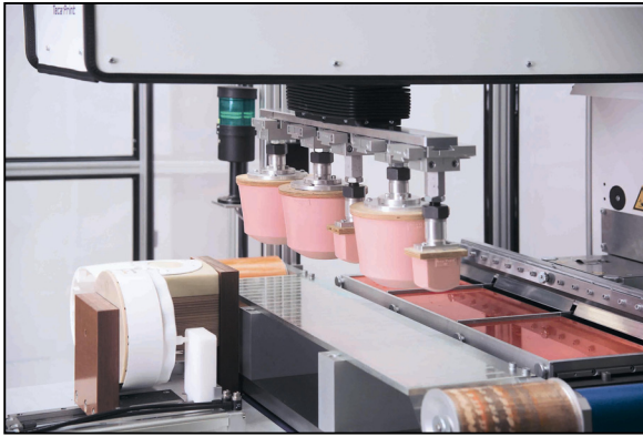
带转换台和移印头清洗设备的 TPX 550 - 可在两个水平面打印
