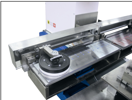
TPX 552 - 2 色打印 - 以及侧面墨杯结构
